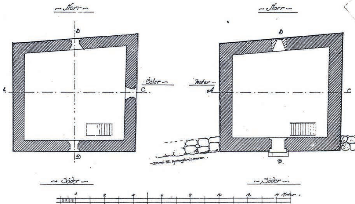
Figur 5. Uppmätning av förrådsboden/tiondeboden upprättad av Sigurd Curman i januari 1907, troligen i samband med att byggnaden skulle inkorporeras i den nya prästgården. Längst ned till höger syns hur grunden till den gamla kyrkogårdsmuren ansluter till byggnadens södra mur. Upplandsmuseets topografiska arkiv.
