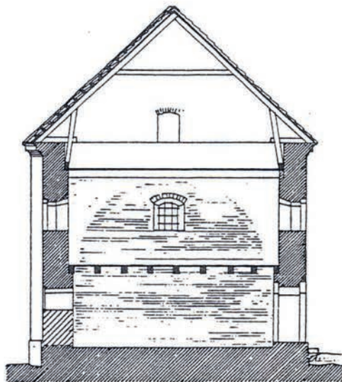
~ Sektion B-D ~
