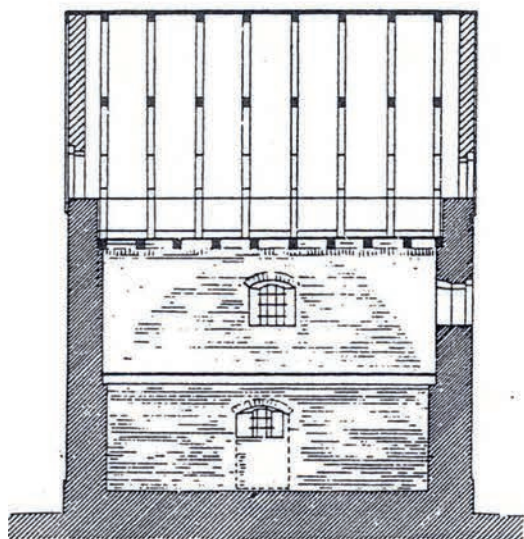
~ Sektion A-C ~
